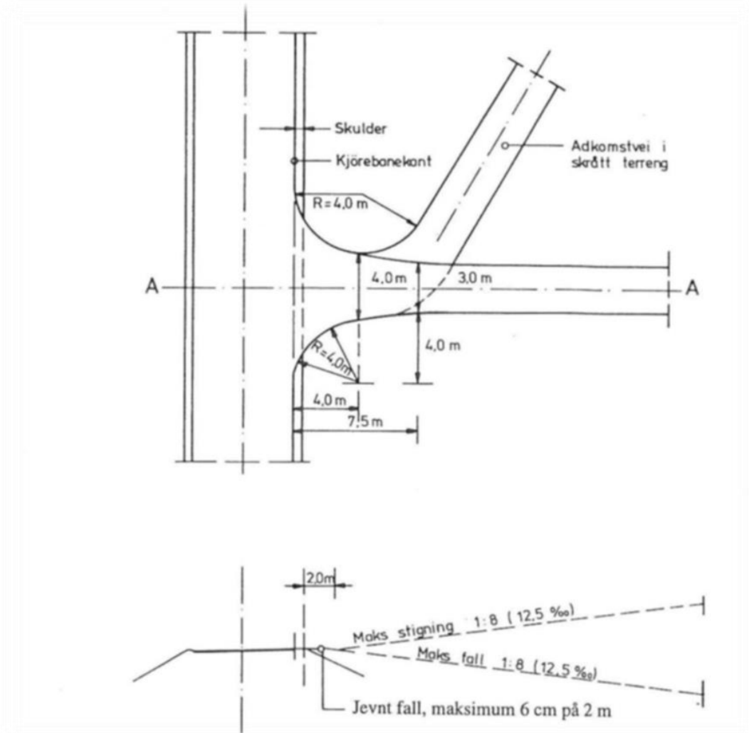
Profil: A-A
